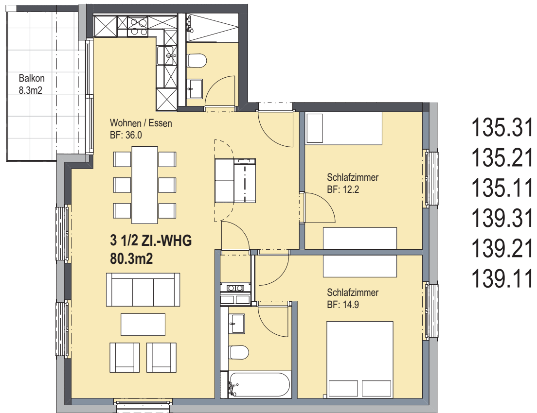
Typ 8 Haus A und B 1.-3.OG 3.5-Zimmerwohnung West
