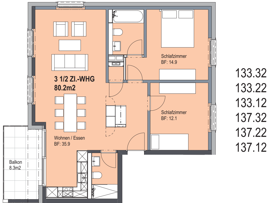
Typ 5 Haus A und B 1.-3.OG 3.5-Zimmerwohnung Ost
