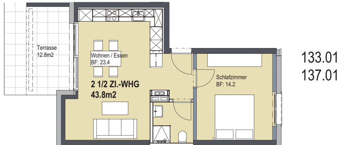
Typ 2 Haus A und B EG 2.5-Zimmerwohnung
